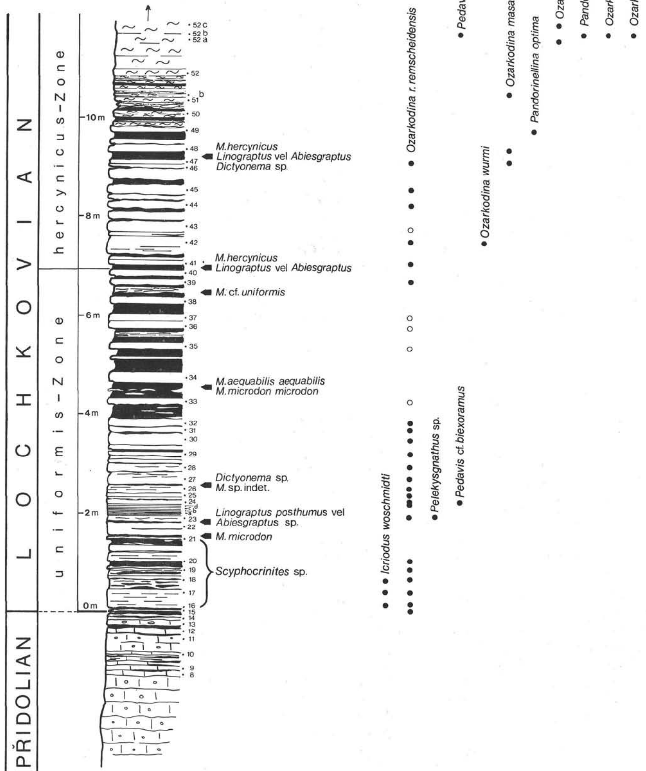
Fig. 13: The Přidolian to Lochkovian section Oberbuchach 2. After H. JAEGER & H. P. SCHÖNLAUB in press (modified).
