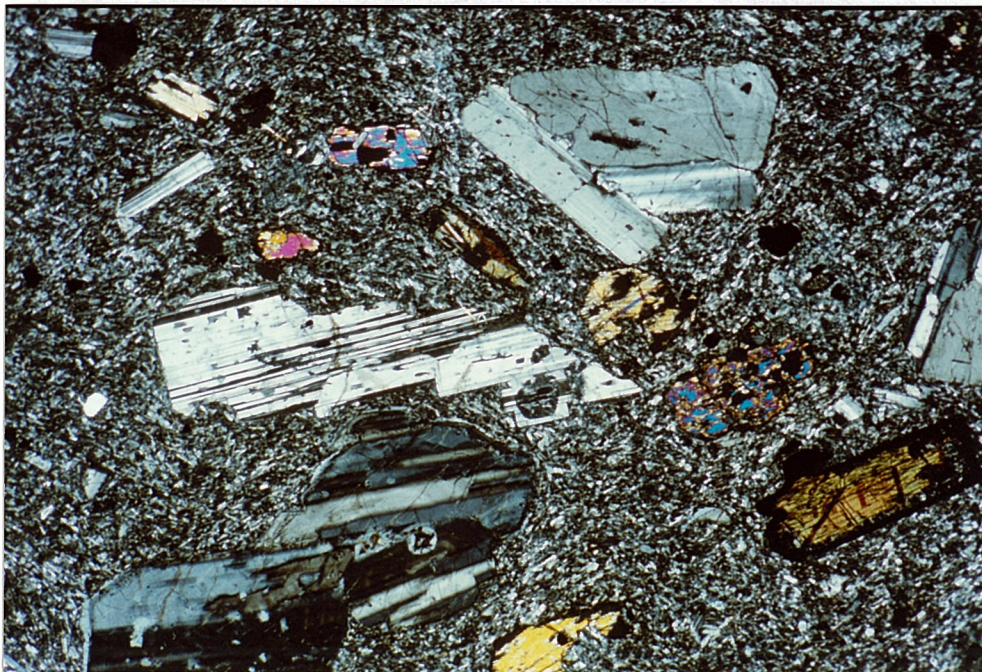
Abb. 11 Probe Nr. 40 25-fach gekr. Nicols
