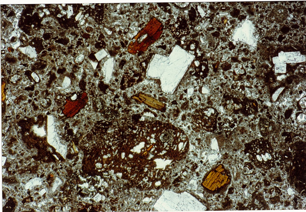
Abb. 38 Probe Nr. 55 25-fach, gekr. Nicols
