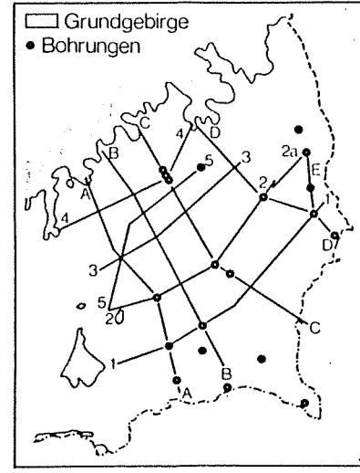
Abb. 60: Geologische Schnitte durch das Oststeirische Tertiärbecken mit Position der miozänen Vulkanitmasse (aus EBNER et al. 1986).
