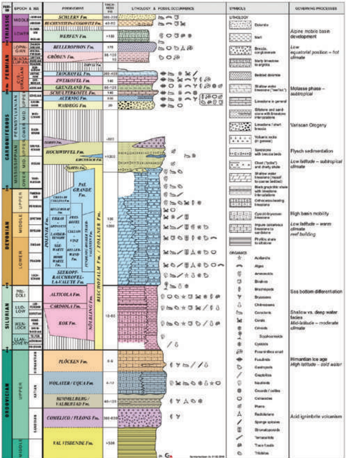
Fig. 1 - Stratigraphic subdivision of the Carnic Alps including governing processes. © Hans Peter Schönlaub. - Schema stratigrafico delle Alpi Carniche con indicati i principali processi che ne hanno governato l'evoluzione. © Hans Peter Schönlaub.
