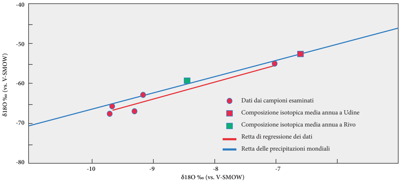
Fig. 7 - Grafico che pone in relazione gli isotopi dell'Ossigeno e dell'Idrogeno nei campioni di ghiaccio analizzati e nelle precipitazioni a livello mondiale (CRAIG 1961; da FLORA et al. 2004). - Graph relative to the isotopes of oxygen and hydrogen in the analyzed ice samples and in the global precipitation (CRAIG 1961; from FLORA et al. 2004).
