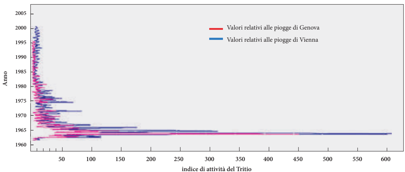
Fig. 8 - Grafico relativo ai valori di attività del tritio nelle precipitazioni delle stazioni di Vienna e Genova, calcolati al 2003 (dati GNIP: Global Network on Isotopes in Precipitations). - Graph relative to the Tritium activity in the precipitations of Wien and Genova, calculated for 2003 (data GNIP: Global Network on Isotopes in Precipitation).
