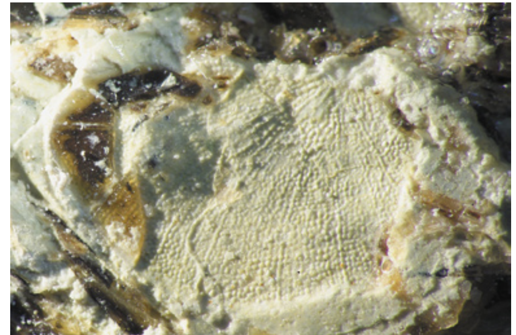
Abb. 8: Aeoliscus apscheronicus (LEDNEV, 1914); Badenium, Mittel-Miozän; St. Margarethen im Burgenland, Steinbruch der Fa. Kummer; Operculum-Abdruck; NHMWien 1976/1837/63, Ausschnitt aus Abb. 3, 13,2 x natürl. Größe. – (NHMWien). Foto: E. HÖCK.
