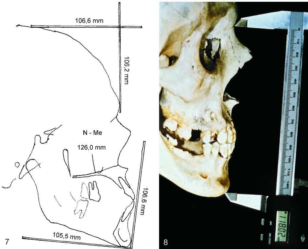
Abb. 7, 8: (7) Fernröntgendurchzeichnung mit Kontrollwinkel 100x100 mm und resultierende Vergrößerung des Röntgenbildes. (8) Elektronische Schiebelehre an Nasion-Menton zur Kontrolle des Vergrößerungsfaktors.
