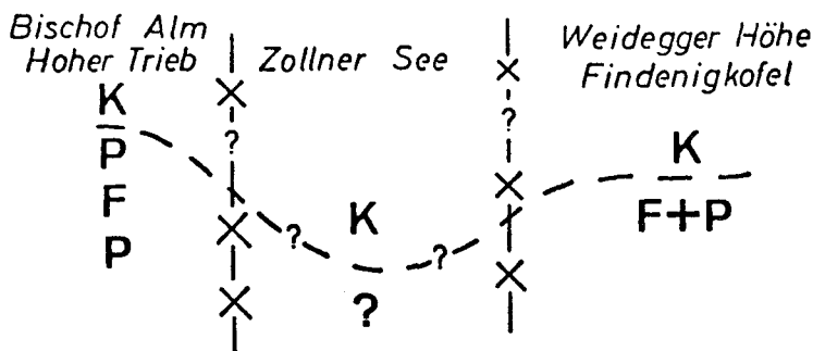
Abb. 2: Faziesverteilung im Silur und Gedinne, schematisch (K = Kieselschieferfazies, P = Plöckener Fazies, F = Findenigentwicklung).
