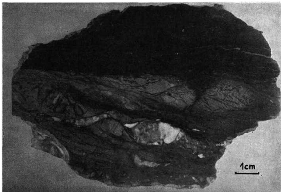
Abb. 5: Sedimentärer Kontakt zwischen Kalken des toIIz (unten) und Hochwipfelkarbon (oben) (Anschliff).
