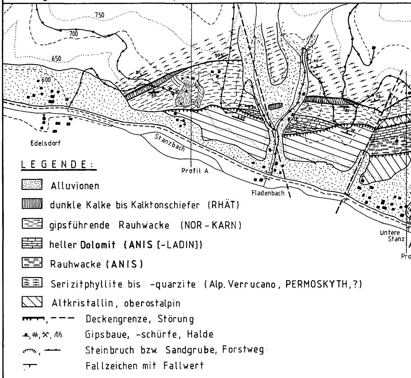
Abb. 1. Geologische Karte.
